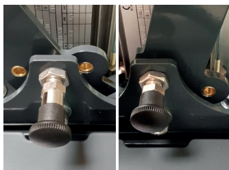
Arretierung mit Rastbolzen (Sonderzubehör)
