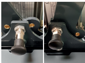
Arretierung mit Rastbolzen (Sonderzubehör)
