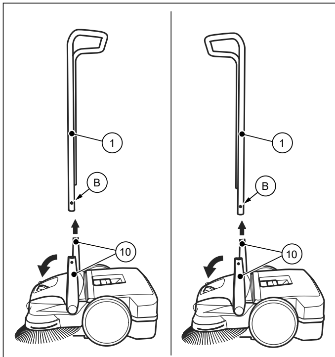
Abb. 9: Schiebebügelmontage
