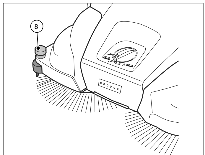
Abb. 6: Niederhalterereinstellung
