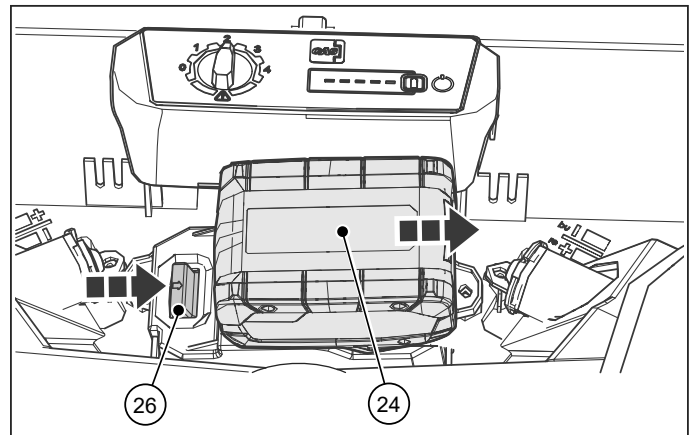
Abb. 10: Akku entnehmen
