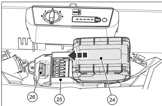
Abb. 4: Akku einbauen
