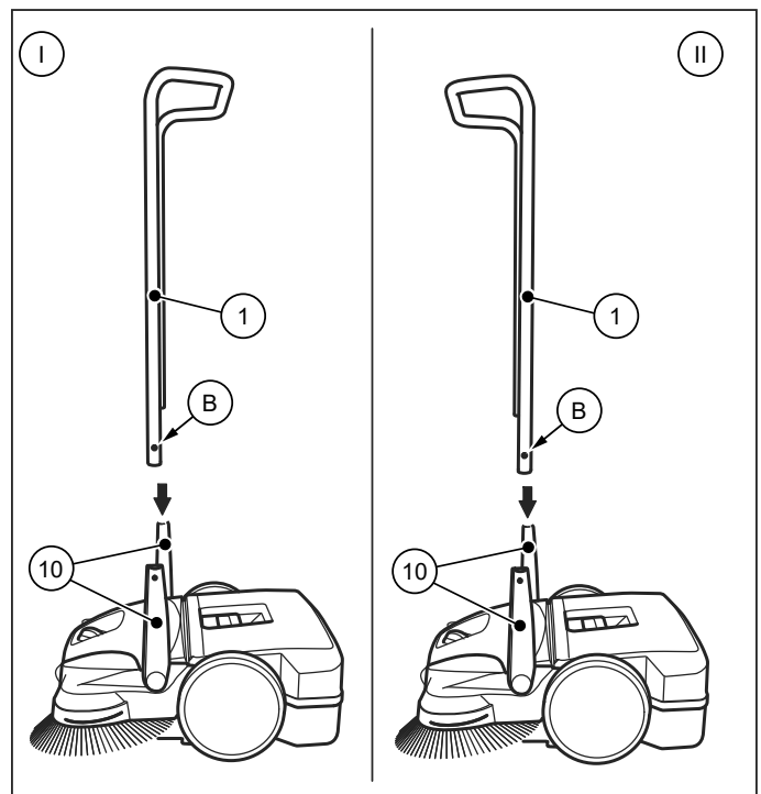
Abb. 3: Schiebebügelmontage
