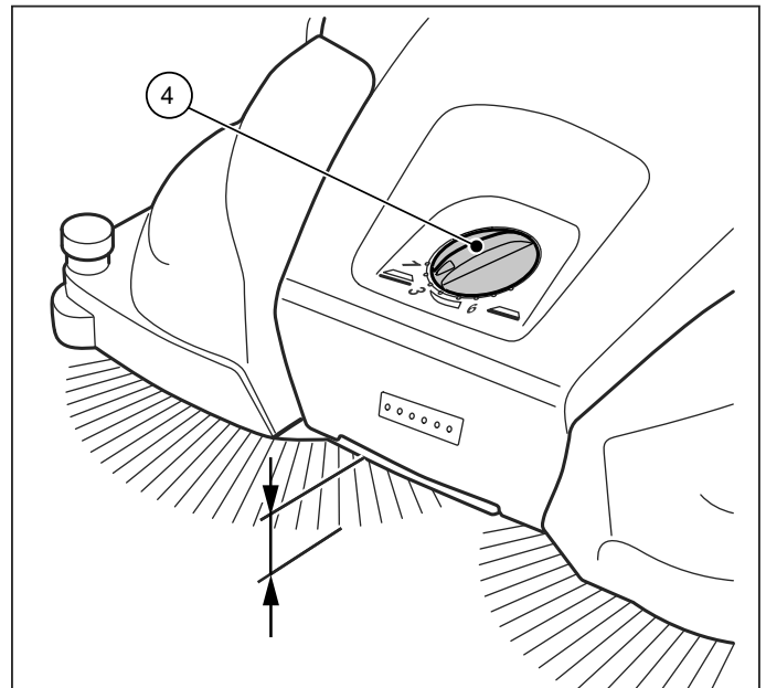
Abb. 5: Höhenverstellung Tellerbesen
