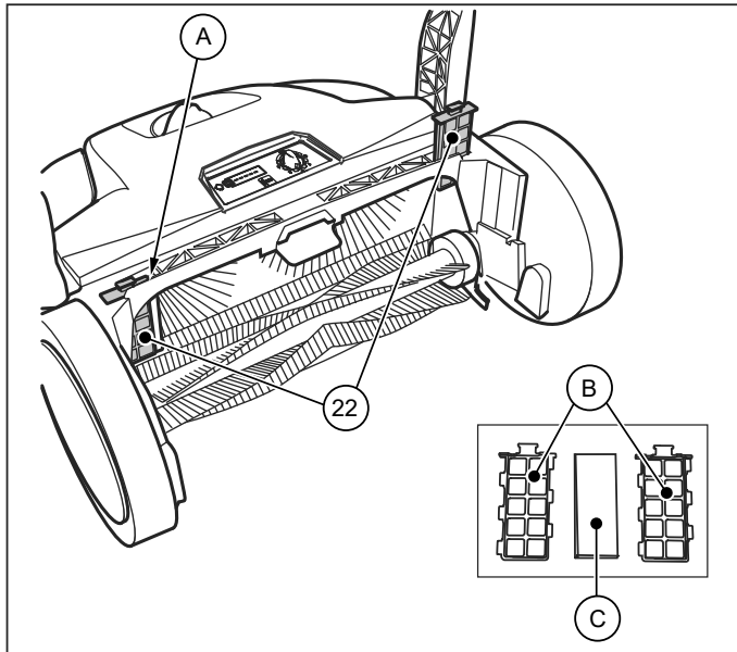
Abb. 8: Staubfilterentnahme
